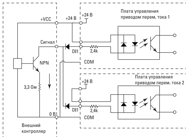
Рис. 3-9. Способ разводки при утечке на клеммах DI нескольких преобразователей частоты
