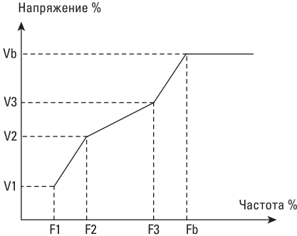
V1-V3: 1-й, 2-й, 3-й проценты напряжения многоточечной кривой V/F Vb: номинальный ток двигателя F1-F3: 1-й, 2-й, 3-й проценты частоты многоточечной кривой V/F Fb: номинальная рабочая частота двигателя
