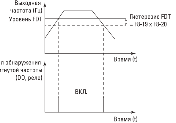
Рис. 6-16. Схема уровня FDT
