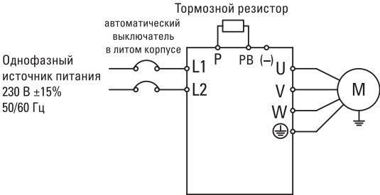
Рисунок 3-2 Стандартное однофазное подключение 0,75–2,2 кВт
