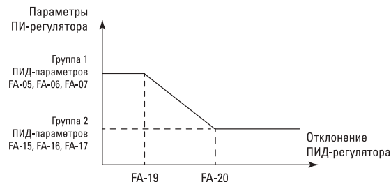
Рис. 6-27. Переключение ПИД-параметров
