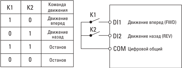
Рис. 6-6. Двухпроводной режим 1
