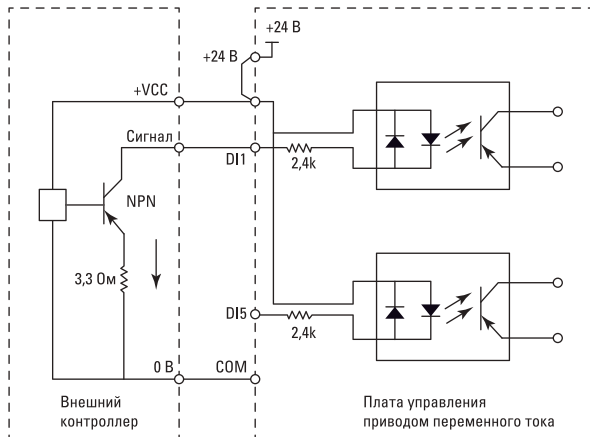
Рис. 3-8. Способ разводки при утечке тока
