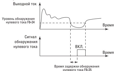
Рис. 6-21. Схема поиска нулевого тока
