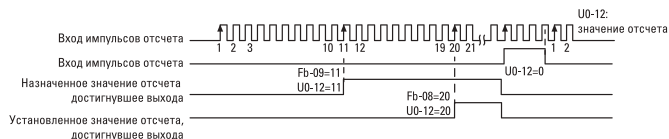
Рис. 6-30. Исходная схема установленного значения отсчета и назначенного значения отсчета
