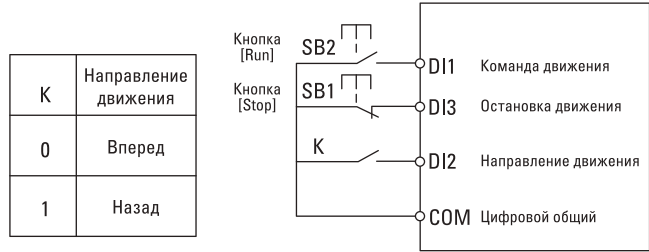
Рис. 6-9. Трехпроводной режим управления 2
