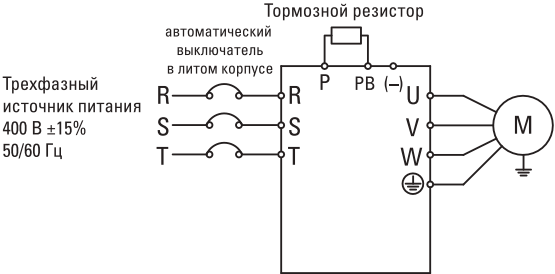
Рисунок 3-3 Стандартное трехфазное подключение 0,75–2,2 кВт
