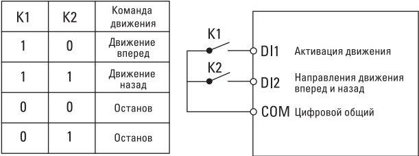
Рис. 6-7. Двухпроводной режим 2
