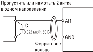
Рис. 3-7. Схема подключения обработки клеммы аналогового входа
