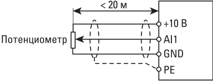
Рис. 3-6. Схема подключения клеммы аналогового входа
