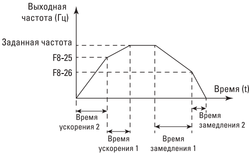
Рис. 6-19. Схема переключения времени ускорения/замедления
