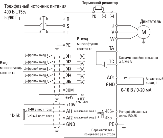
Рис. 3-5. Режим проводки контура управления преобразователя частоты
