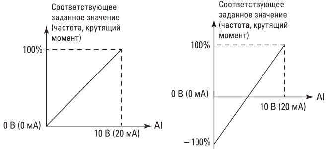
Рис. 6-10. Соответствующие соотношения между аналоговым опорным сигналом и заданными значениями
