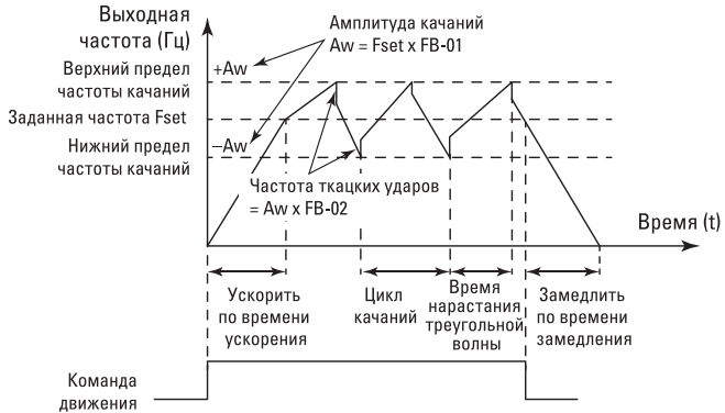
Рис. 6-29. Схема частоты качаний
