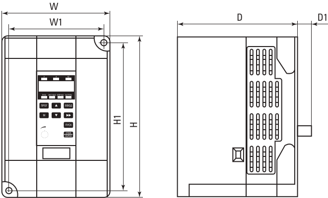
Рис. 7-1. Внешний вид пластмассовой конструкции и монтажные размеры VECTOR-75
