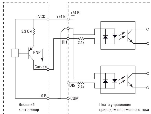
Рис. 3-10. Соединение (PNP). Проводка выходной клеммы управляющего сигнала
