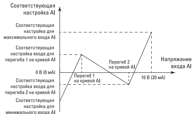
Рис. 6-33. Схема кривой 4 и кривой 5
