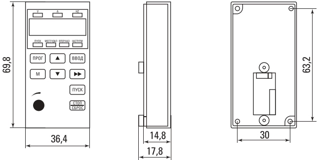
Рис. 7-2 Габаритные размеры интегрированной клавиатуры
