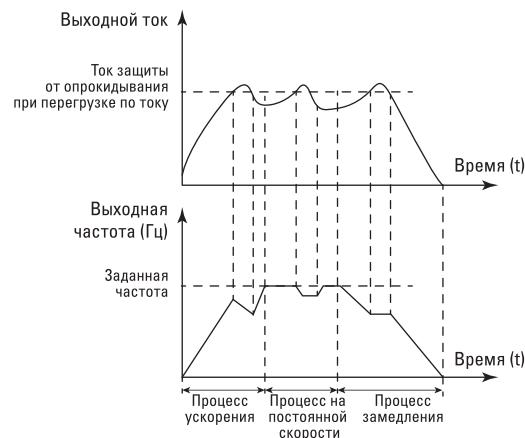
Рис. 6-24. Схема защиты от опрокидывания при перегрузке по току
