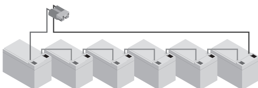
Рисунок 5. Подготовка внешних АКБ
