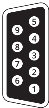
Рисунок 8. Коммуникационный порт RS-232 (коннектор DB-9)
