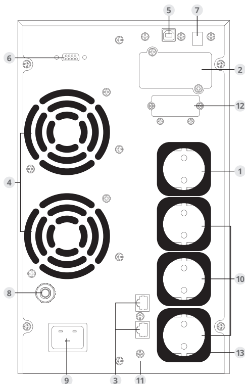
Рис. 3: Вид сзади: ИБП ИМПУЛЬС СТАЙЕР11-2 (2 кВА) и СТАЙЕР11-3 (3 кВА)
