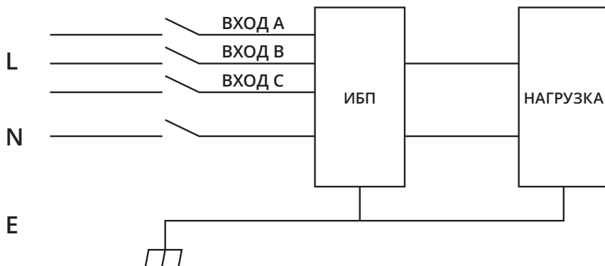
Рис. 2. Правильная конфигурация электропитания
