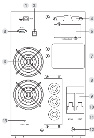
Рис. 1-2: Вид сзади
