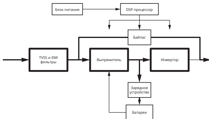
Рис. 1-7: Эко-режим
