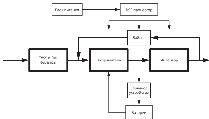
Рис. 1- 8: Режим Self Aging (самотестирования)
