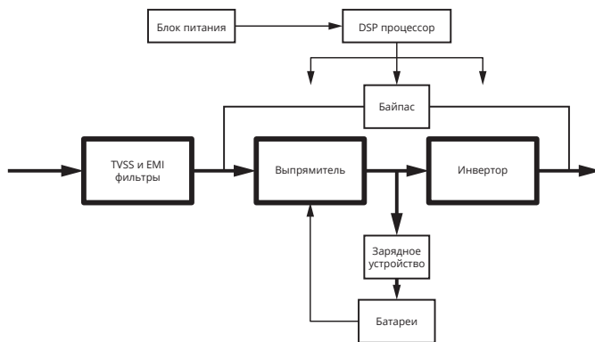
Рис 1-4: Нормальный режим
