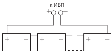
Схема последовательного подключения аккумуляторов к ИБП
