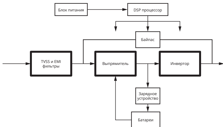
Рис 1-3: Система ИБП
