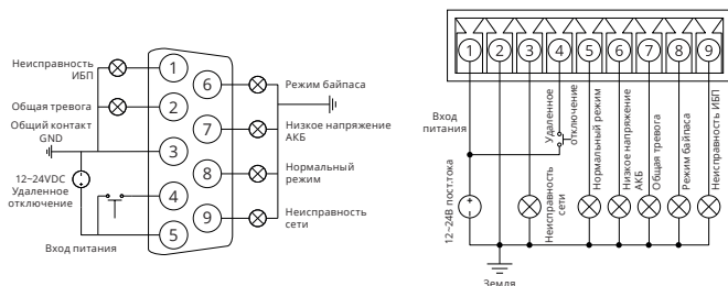
Рис. 5-2: Подключение к внешнему источнику питания
