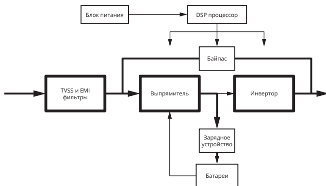
Рис 1-5: Режим байпаса
