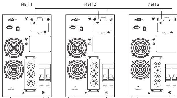
Рис. 2-4: 3 параллельных ИБП
