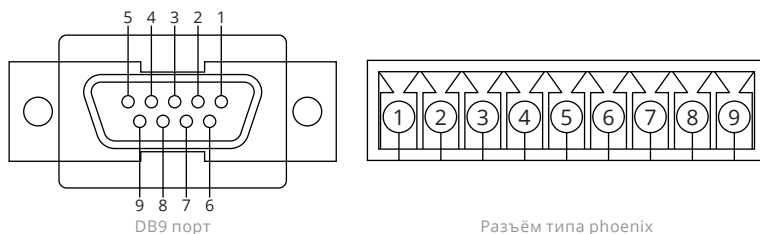
Рис. 5-1: Сухие контакты
