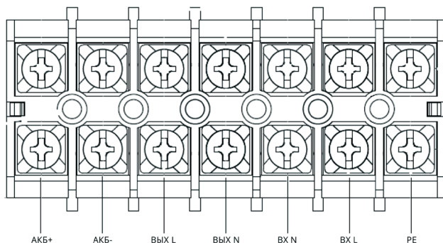
Рис 2- 1: Схема подключения клеммного блока
