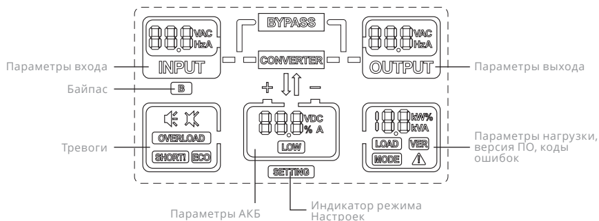
Рис. 3-2: Меню ЖК-дисплея
