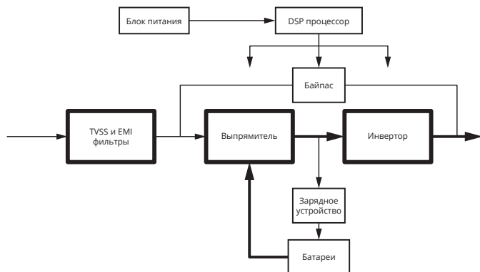
Рис 1-6: Режим работы от АКБ
