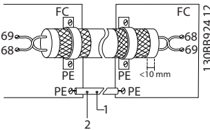
Рисунок 3.10 Кабели из витой пары без клеммы 61
