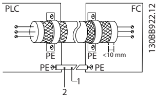
Рисунок 3.7 Экранирующие зажимы на обоих концах
