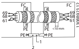
Рисунок 3.9 Кабели из витой пары
