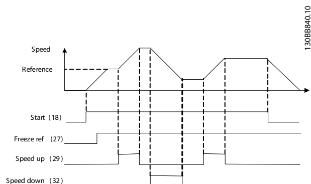
Рисунок 5.1 Увеличение/снижение скорости
