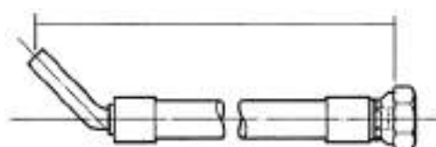
45° standpipe
