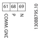
Рисунок 5.2 Подключение сети
