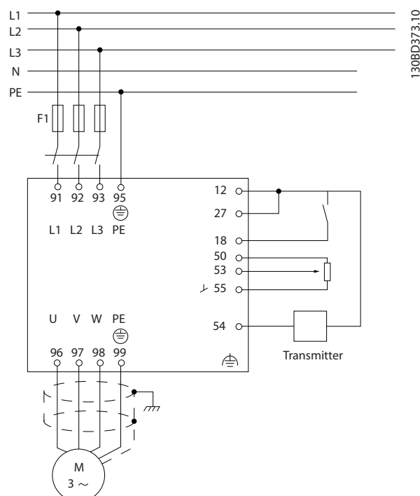
Рисунок 2.25 Двухпроводный датчик
